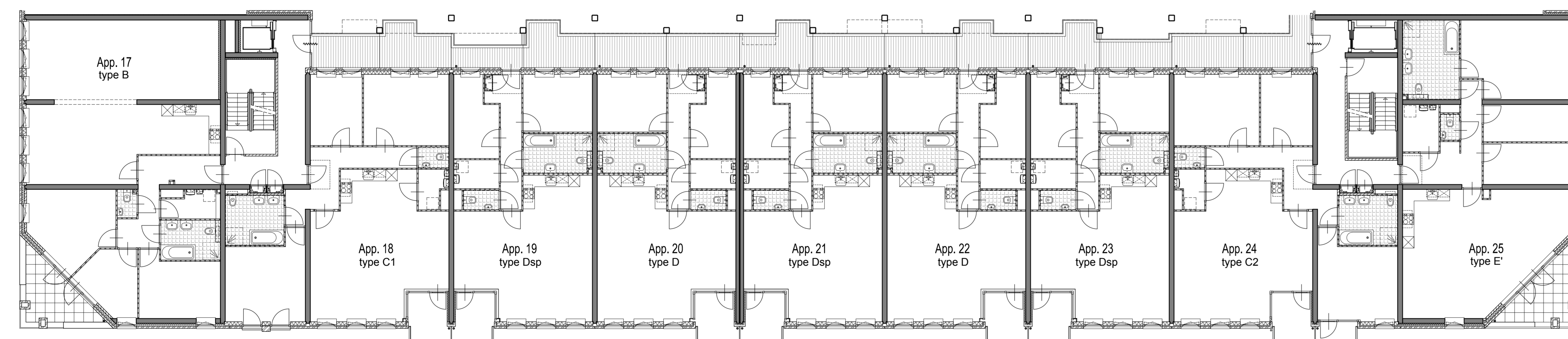
Tweede verdieping (1:200)
