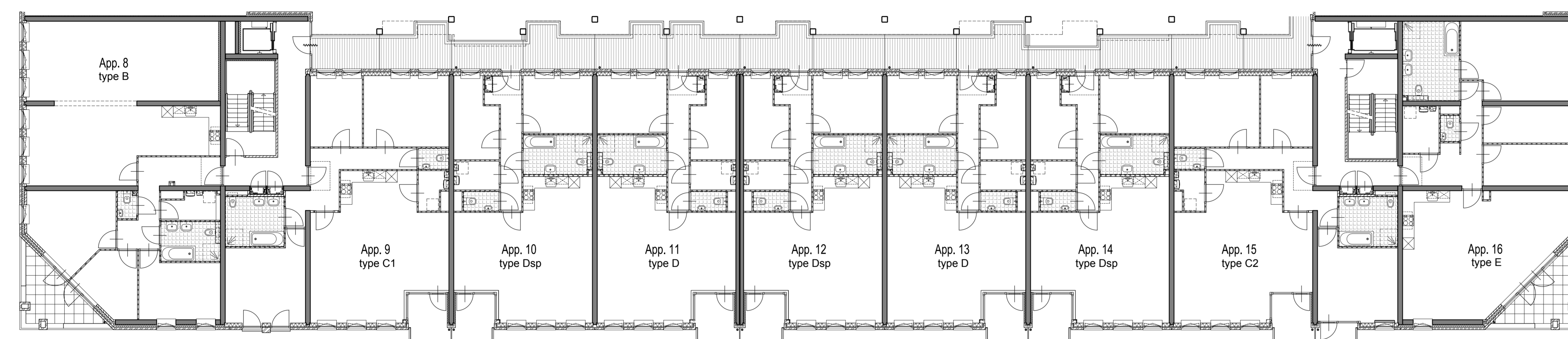
Eerste verdieping (1:200)
